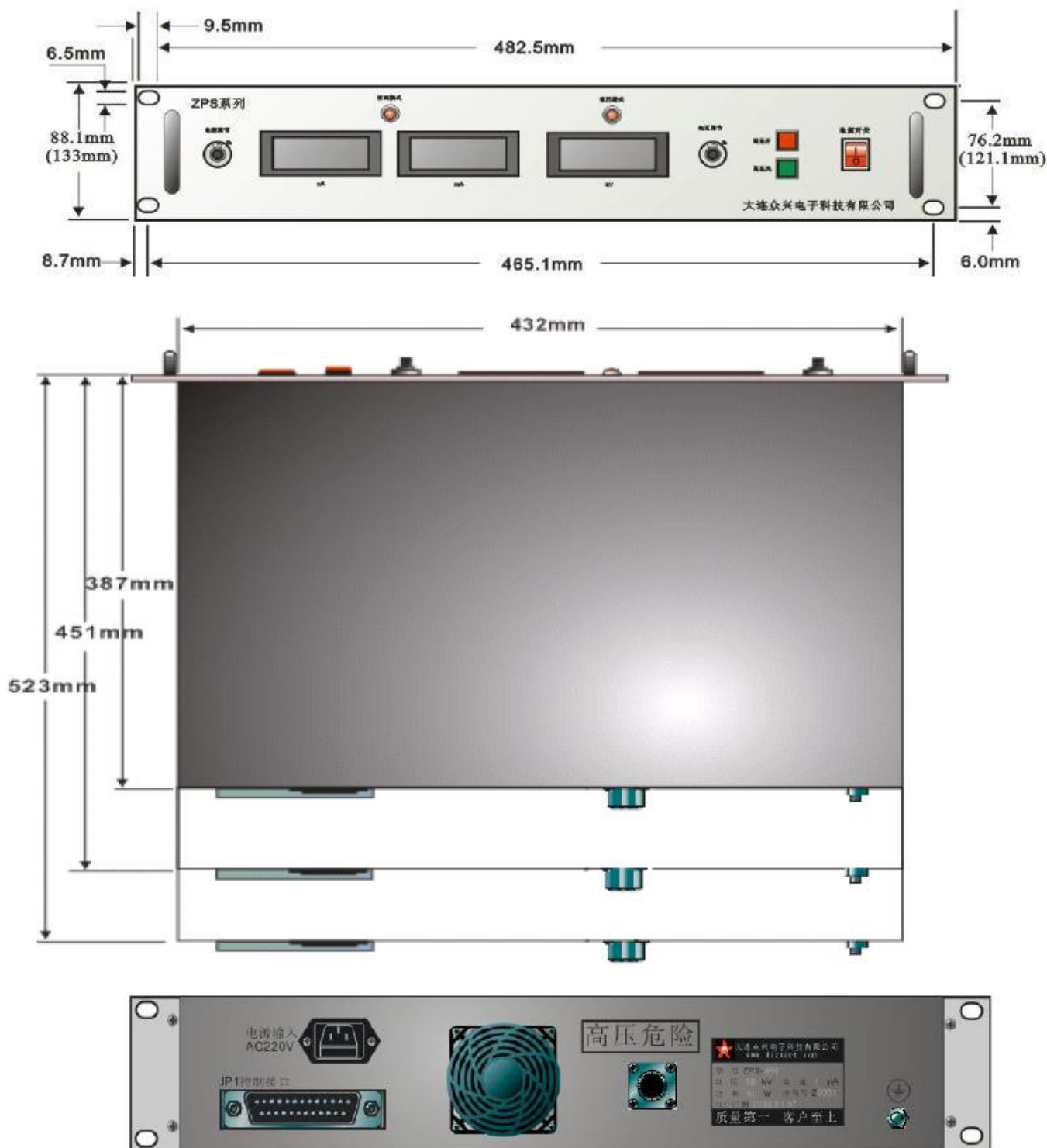
机械尺寸图
